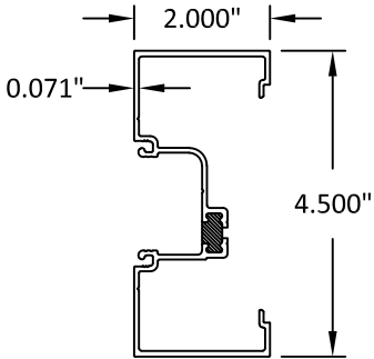
2 MULLION JAMB
