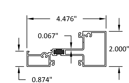
4 HORIZONTAL
